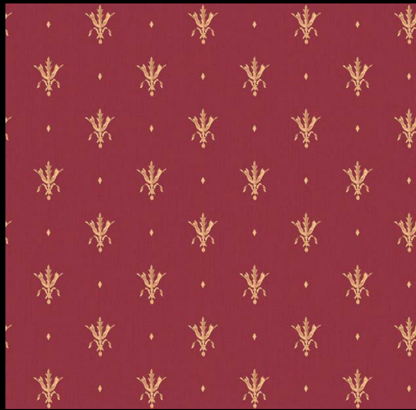
PIAZZATO ORNAMENTALE
